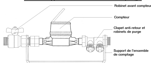
Schéma-type d'un ensemble de comptage
